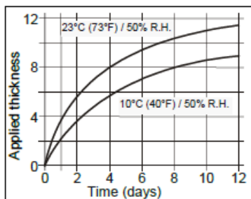
Tabuľka 1: Priebeh vytvrdzovania SikaTack®-Drive
