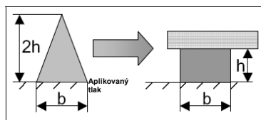
Obr. 1: Stlačenie pásu lepidla do konečnej veľkosti
